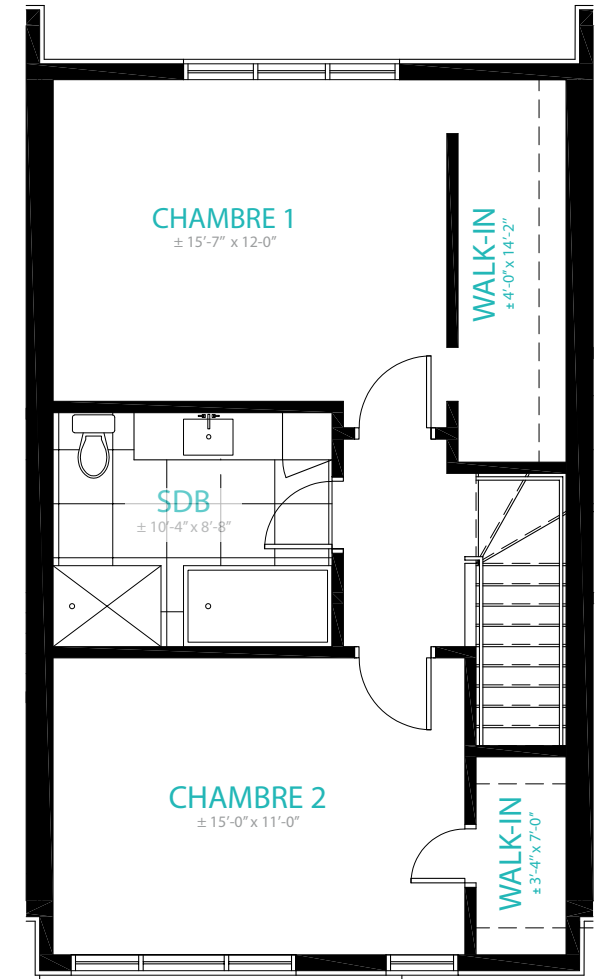
plan type 2 e étage ± xxxx pi ca
